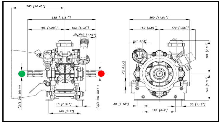
DIMENSIONI D'INGOMBRO - OVERALL DIMENSIONS
